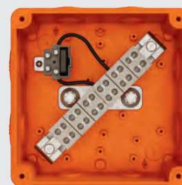
CSATLAKOZÓK ÁTLÓS HELYZETBEN BIZTOSÍTÉKKAL
