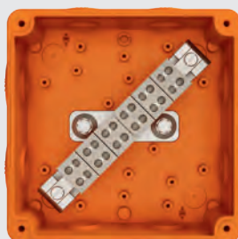
CSATLAKOZÓK ÁTLÓS HELYZETBEN
